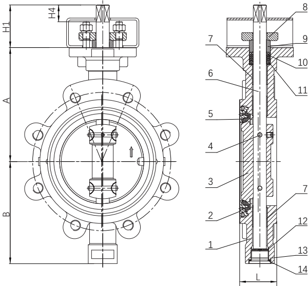
Fig.3645 单夹式
