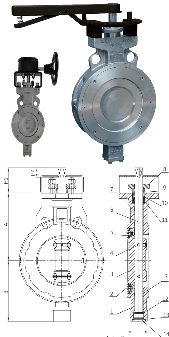
Fig.3635 对夹式
